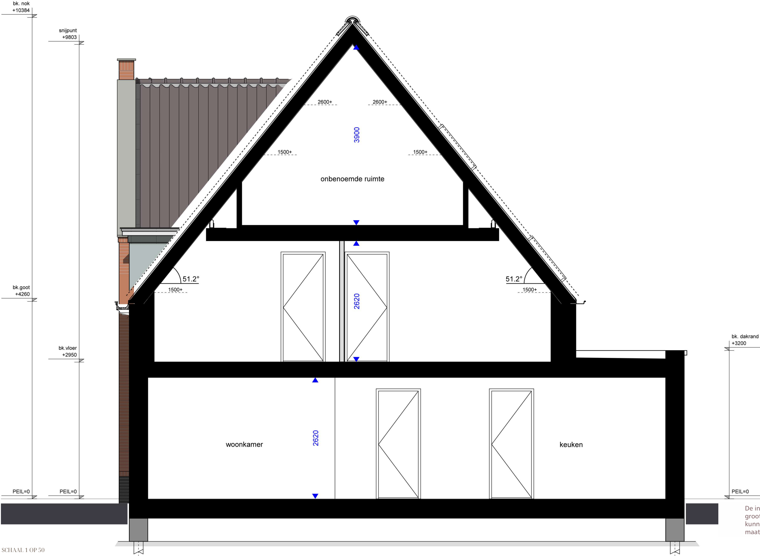
SCHAAL 1 OP 50 Doorsnede
